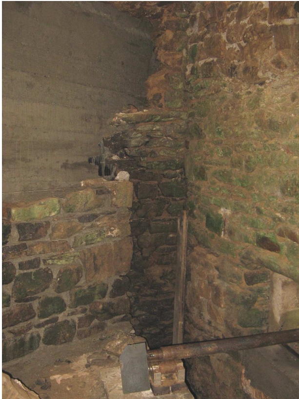
Vue du mur béton coulé et du mur de maçonnerie en cours de réalisation
